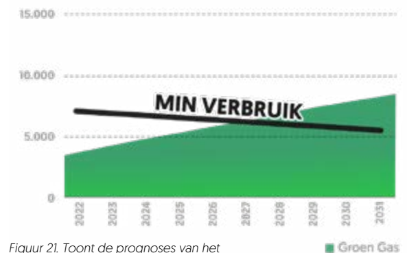
Figuur 21. Toont de prognoses van het opgestelde groen gas productievermogen en het minimale gasverbruik per uur in het Klimaatakkoord scenario.
