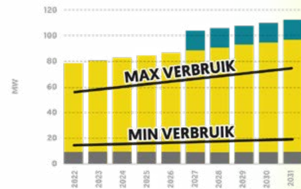
Figuur 22. Prognose van de energietransitie-effecten op het piekverbruik in het Klimaatakkoord scenario ten opzichte van 2020.
