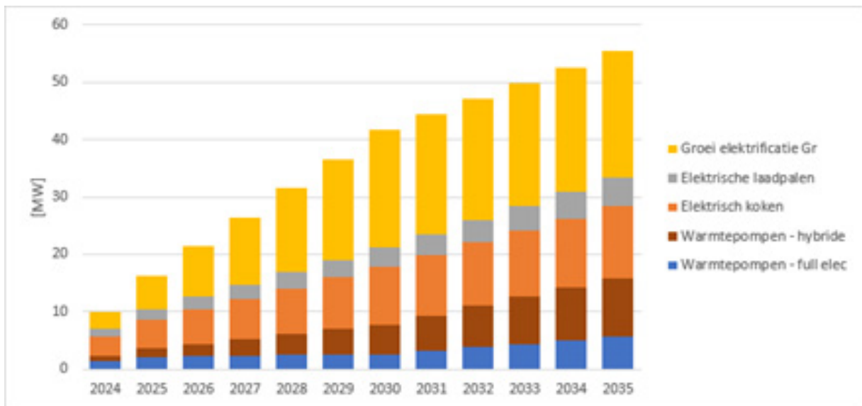
Figuur 20 Prognose van de elektrificatie-effecten op de extra capaciteitsbehoefte van de elektriciteitsnetten in het IA-scenario
