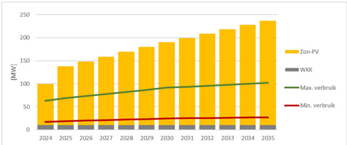
Figuur 19 Prognose van het opgestelde decentrale productievermogen alsook het maximale en minimale elektriciteitsverbruik in het IA-scenario
